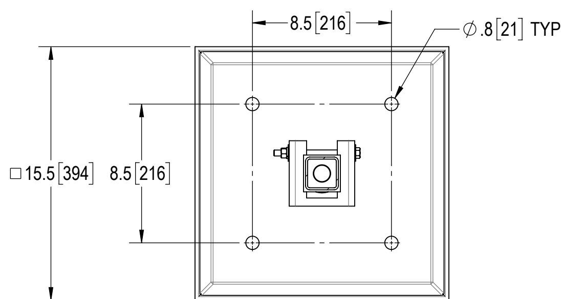
SECTION F-F SCALE 1 : 6
