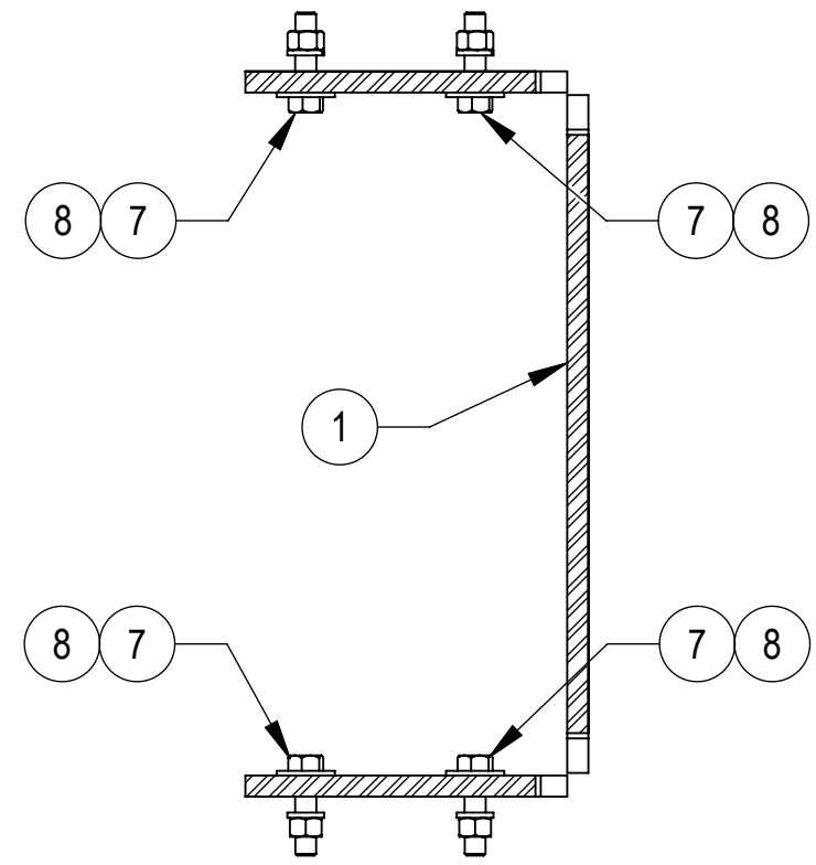
SECTION D-D SCALE 1 : 5
