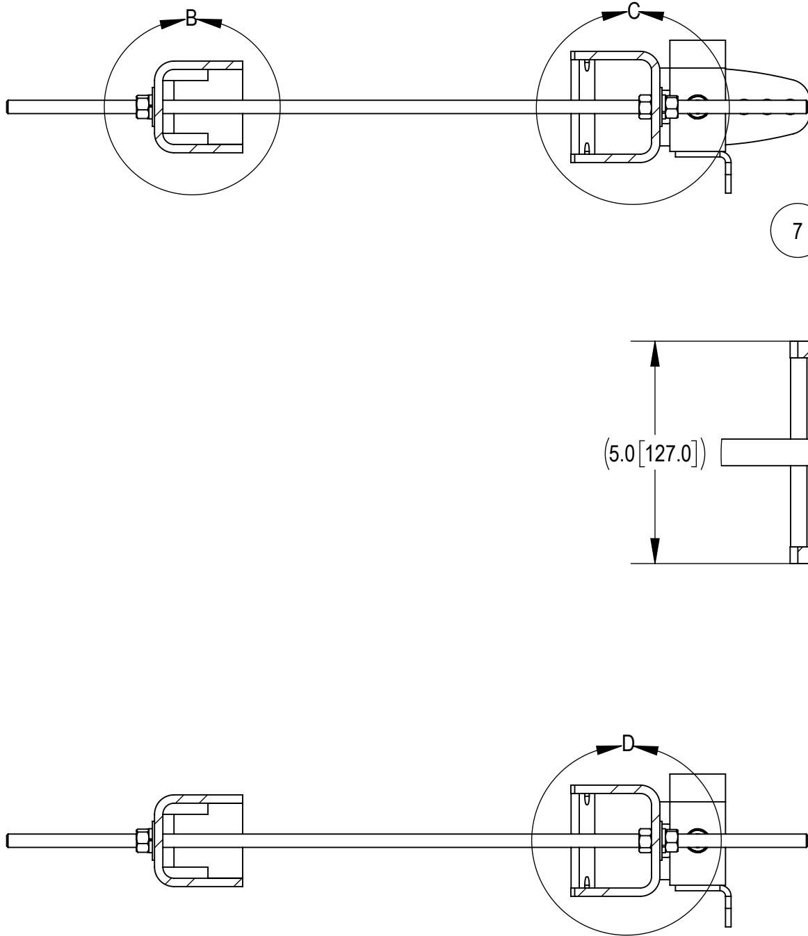
SECTION A-A
